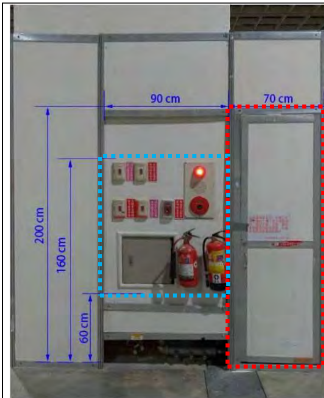
南港 1 館 1 樓展場結構柱隔間牆北側示意圖
