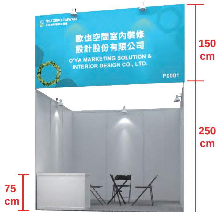
台灣國際淨零永續展-標攤樣式
